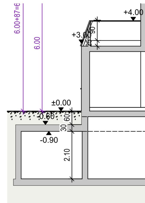
Schnitt Überdeckung TG M 1/100
